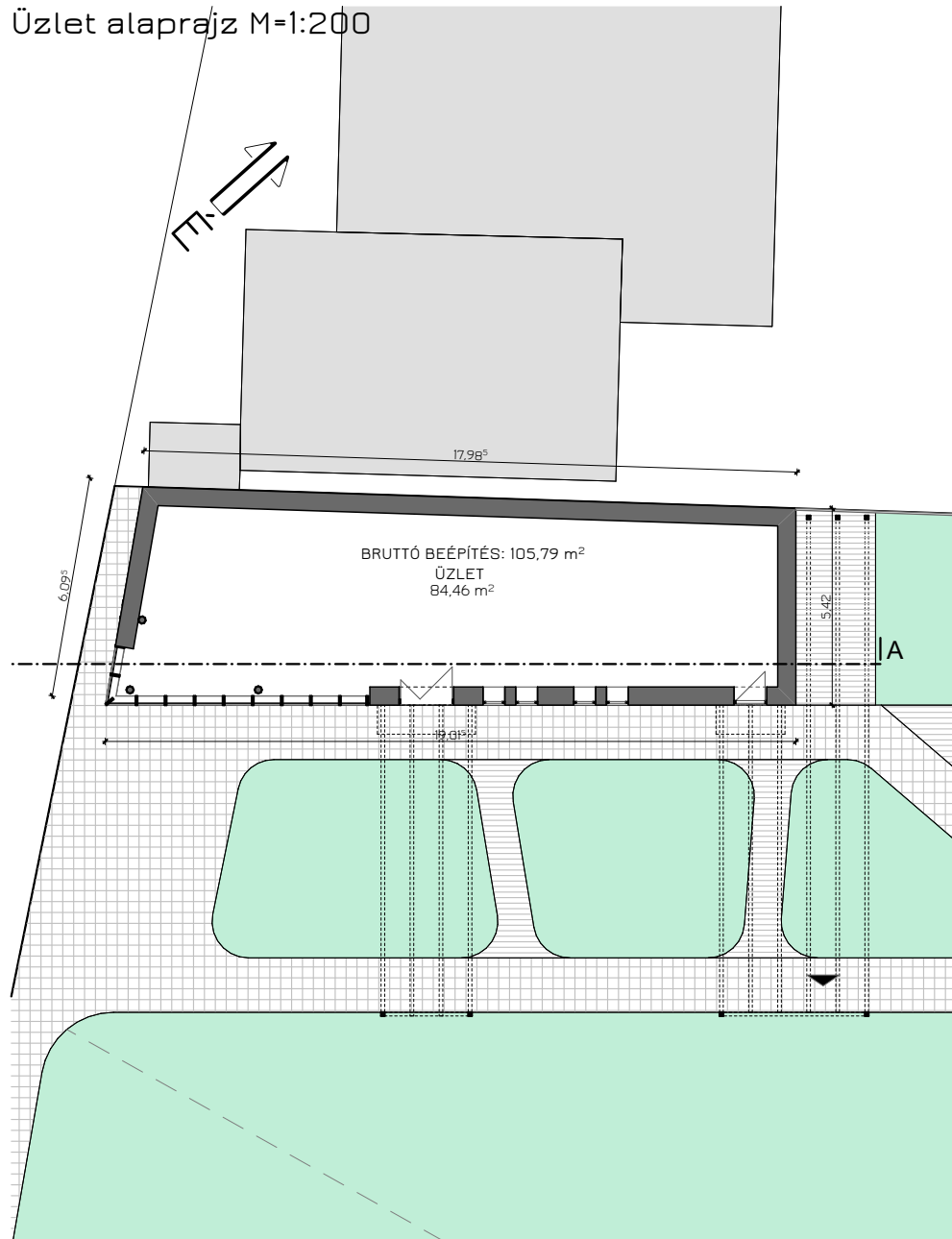
Üzlet/Iroda alaprajz M=1:200
