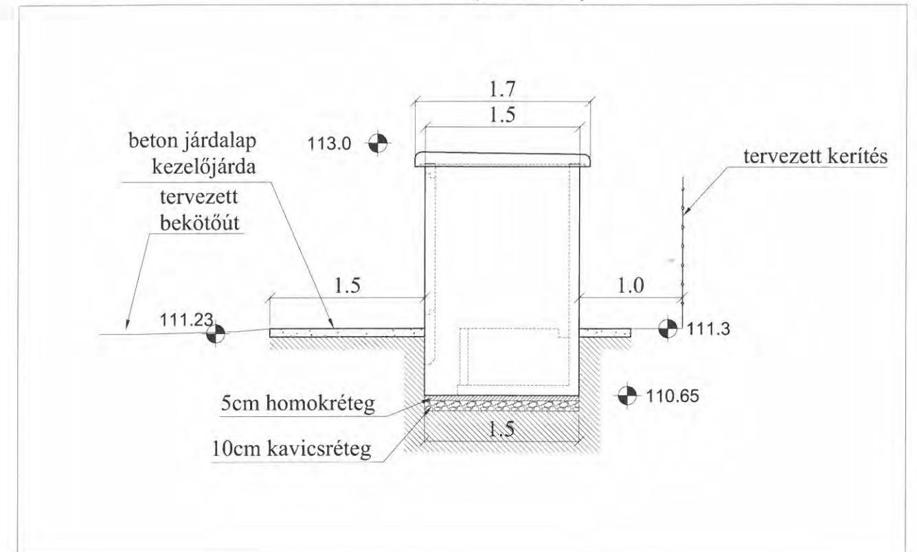
B-B nézet (metszet)
