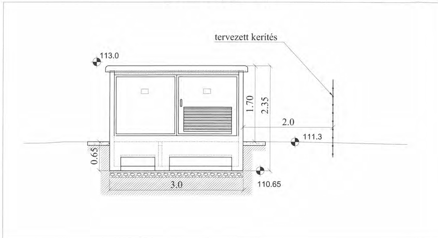
A-A nézet (metszet)
