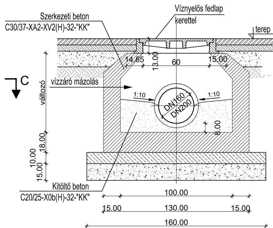
A-A metszet
