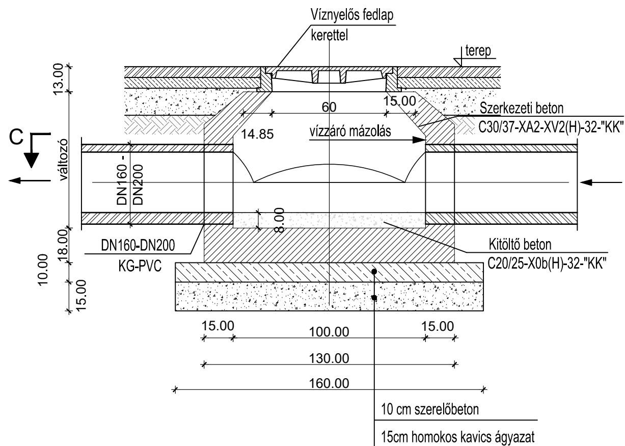
B-B metszet
