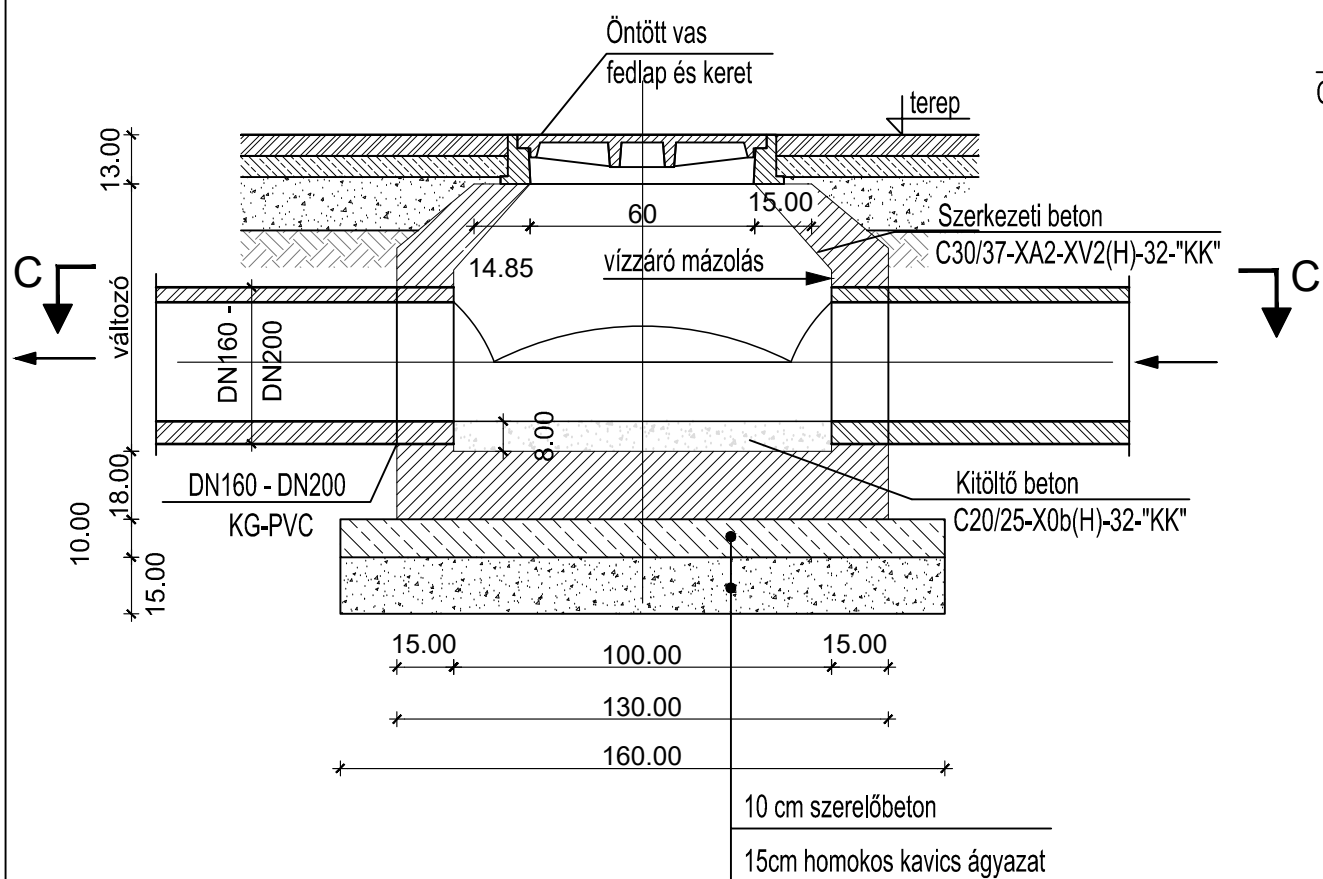
B-B metszet
