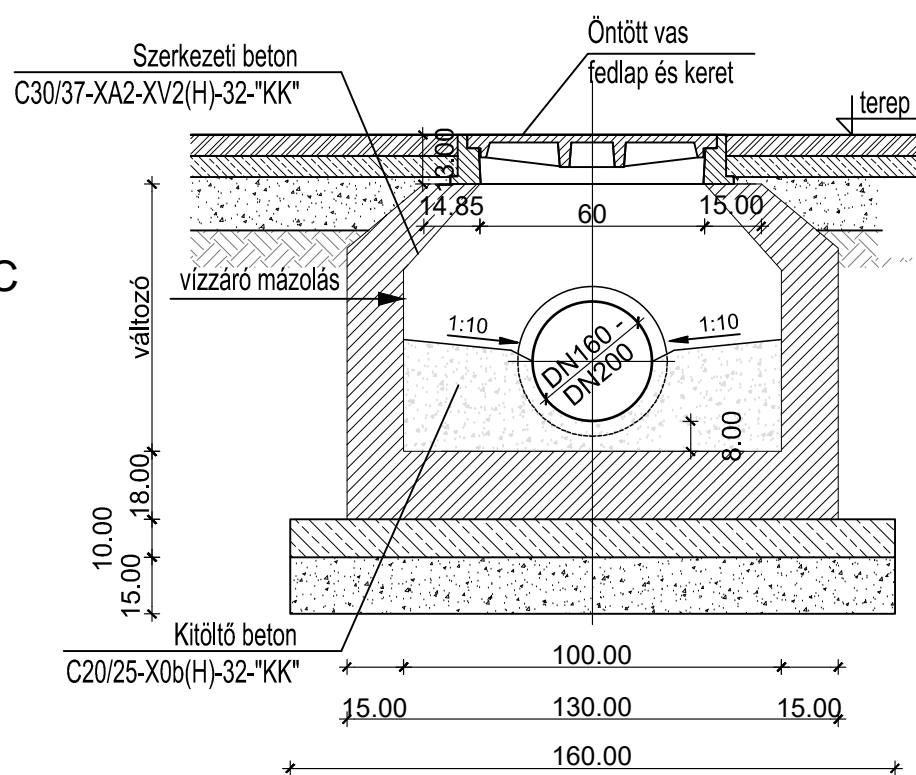
A-A metszet
