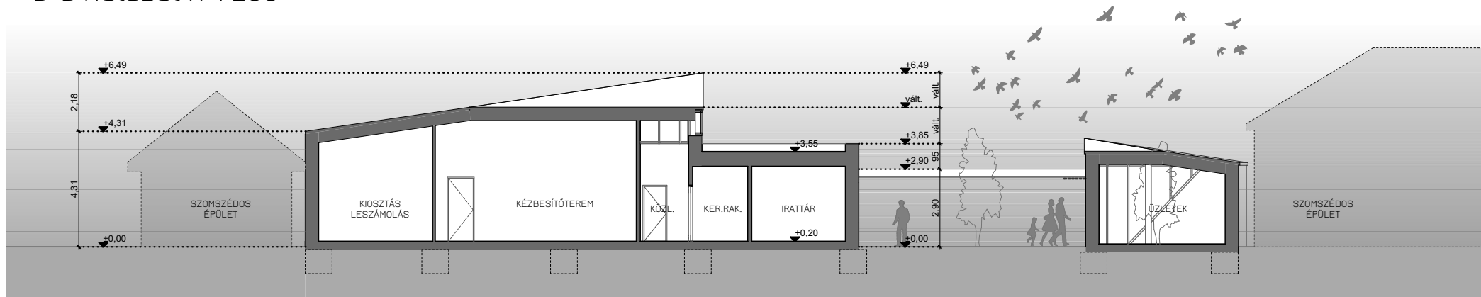
B-B Metszet M=1:200
