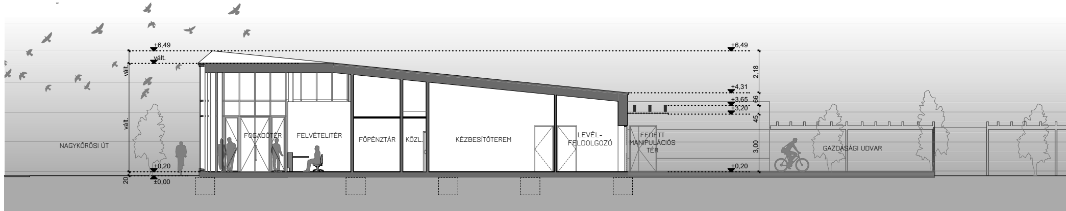
A-A Metszet M=1:200
