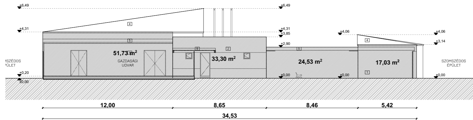
Északkeleti Homlokzat M=1:200
